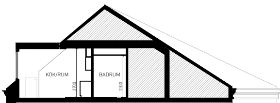
PRINCIPSEKTION SKALA 1:200
