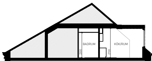
PRINCIPSEKTION SKALA 1:200
