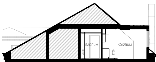
PRINCIPSEKTION SKALA 1:200
